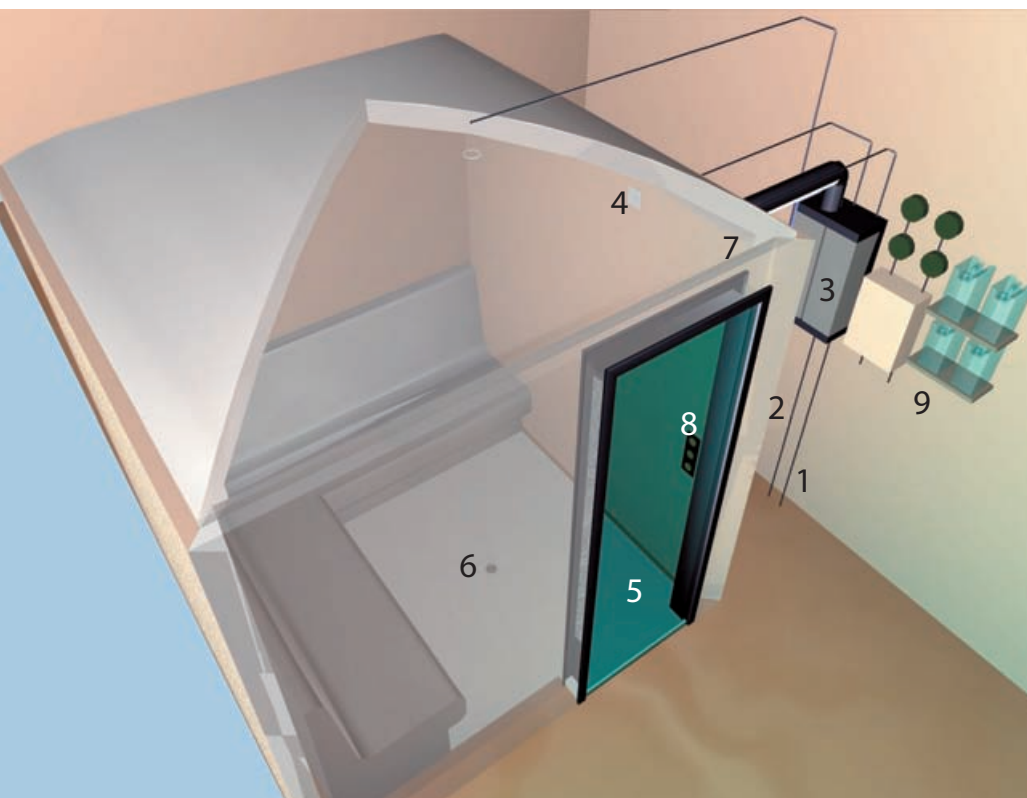
Elementi di un bagno turco.
